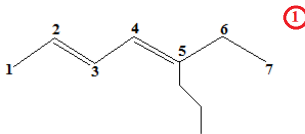
-d- 5-propylhept-(2,4)-diène.....
