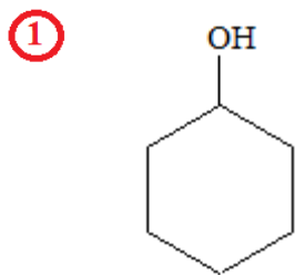
-c- Cyclohexanol.....
